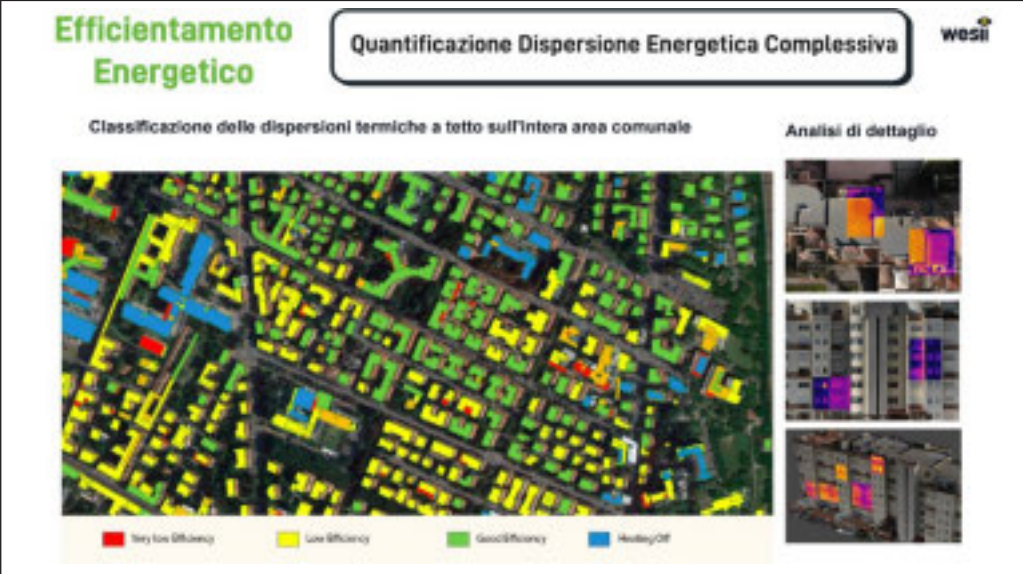
Un modello di rilevamento che assegna colori diversi al fenomeno della dispersione termica
